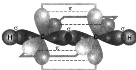
Зв'язки в молекулі етіну
