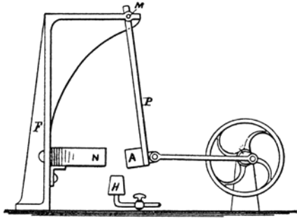
Рис. 4.1. Термоелектричний двигун Тесли 1886 року:
